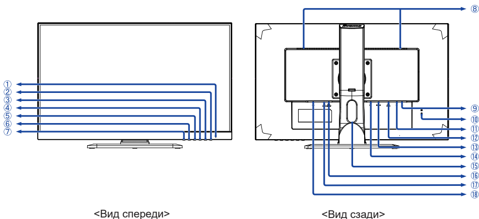
<Вид спереди>
