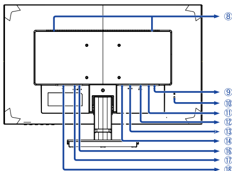
<Вид сзади>
